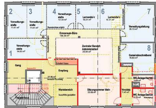
«Haus der Gemeinde»: 1. Obergeschoss
