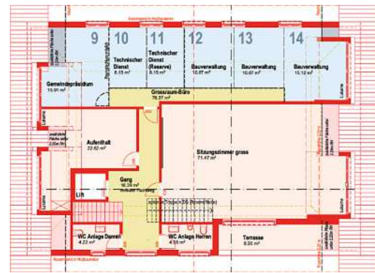
«Haus der Gemeinde»: 2. Obergeschoss
